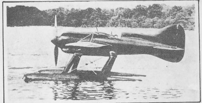
El "Mercurio", del Teniente AL WILLIAMS, un fracaso americano.
